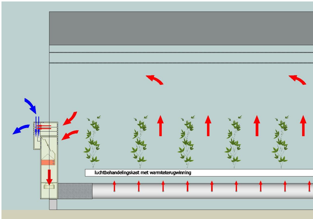
System 4: Schermventilator + verdeelventilator
