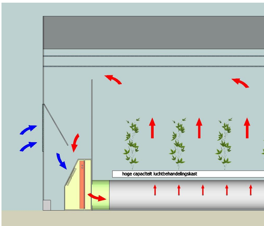
System 8: Hoge capaciteit LBK
