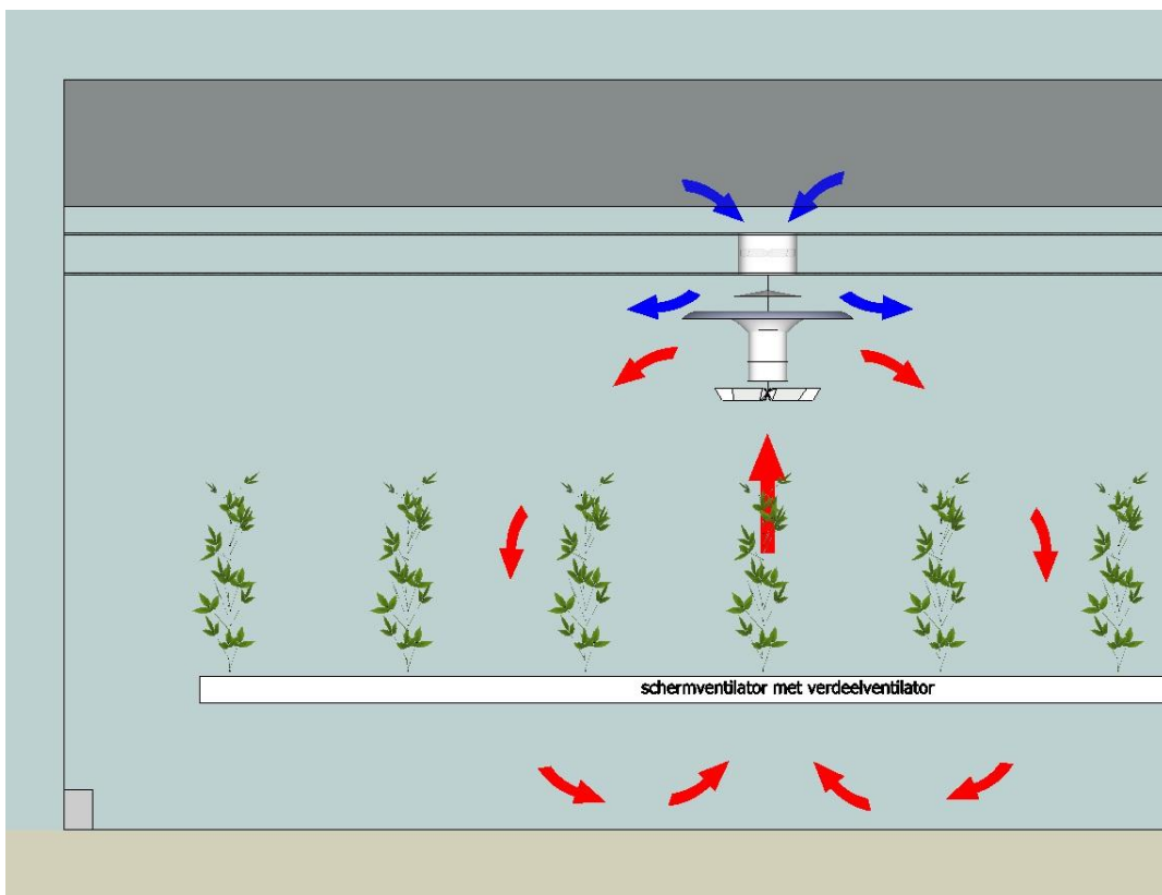
System 4: Schermventilator + verdeelventilator
